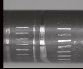
Falso Brinell em um eixo em que um rolamento de rolos cilíndrico foi montado
