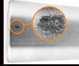
Corrosão localizada por arco elétrico
