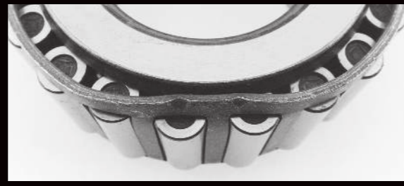
Deformação do porta-rolos
