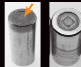
Dano por calor no encosto e extremidade do rolo
