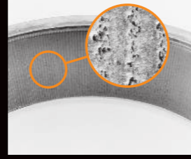
Estriamento por arco elétrico
