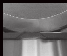
Encosto do anel interno fraturado
