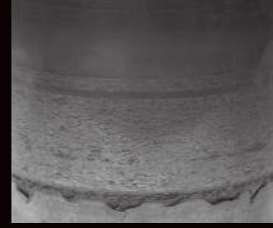
Rolamento autocompensador de rolos com desgaste adesivo
