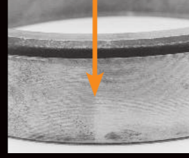
Marca por ponto alto no mancal
